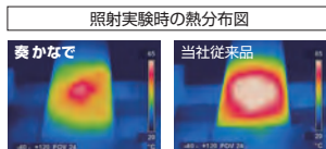
測定機器: チョー製 サーマビジョン CPA-8000 商品色: モカブラウン(WBR) ©同時に照射を開始し、1時間半後に撮影
